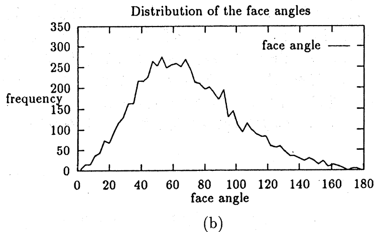
図 7. Laplacian スムージングによる面の交角の変化 (文献 [15] より)
