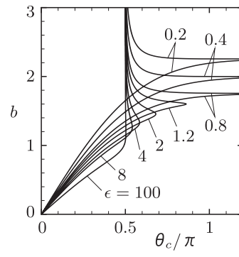
Fig. 14. Dimensionless impact parameter b vs. \theta_c .
