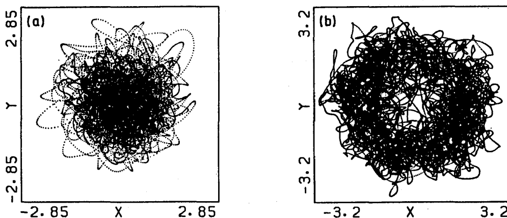
図1. ひとつの局所場の複素平面上のポートレート
