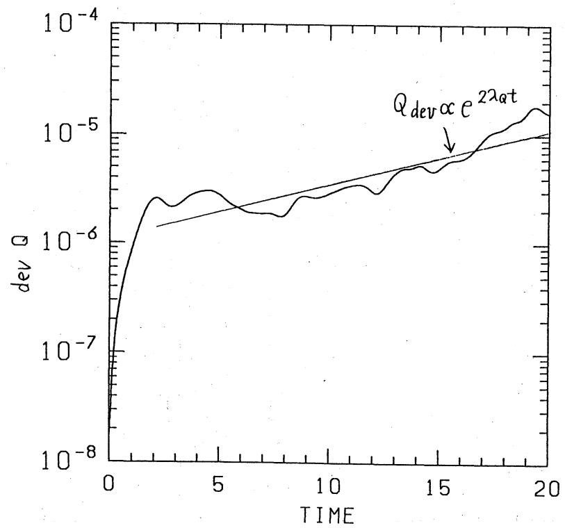
図9 異なる擾乱の時間発展
