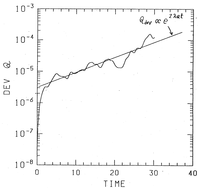
図6 Q_{\text{dev}} \equiv \|\Delta u\|_Q^2 の時間変化, \lambda_Q = 0.058
