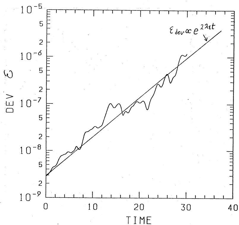
図5 \varepsilon_{\text{dev}} \equiv \|\Delta u\|_E^2 の時間変化, \lambda_\varepsilon = 0.093
