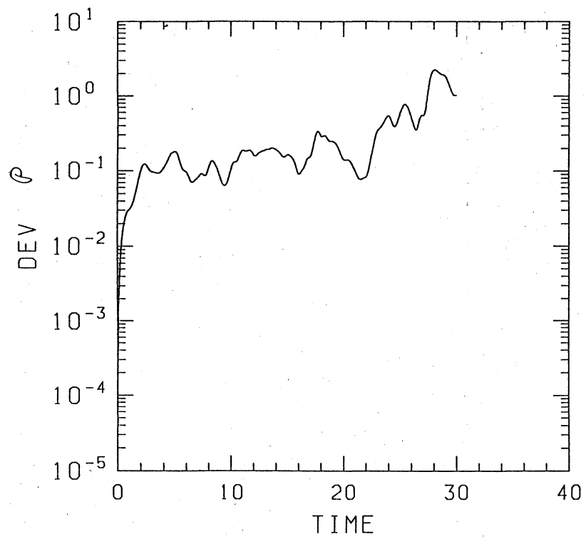
図7 P_{dev} \equiv |\Delta u|^2 の時間変化
