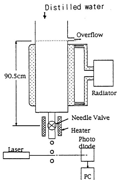
図1 装置の概略。
