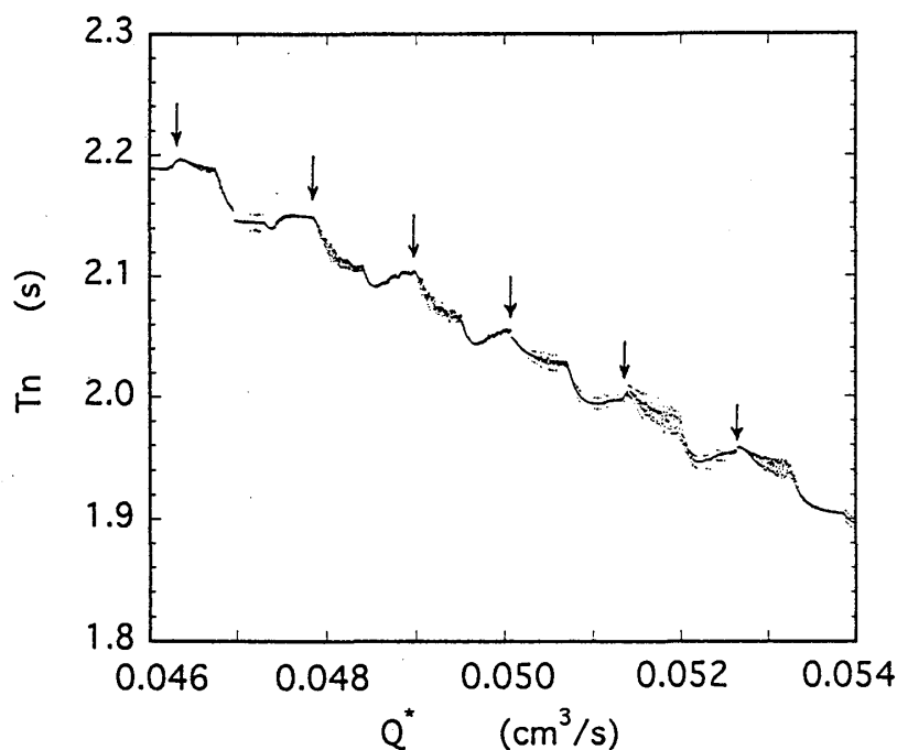
図2 比較的流量の小さな領域での Dripping Spectrum. ↓は安定領域とカオス領域の境界を示す。
