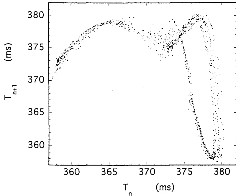
図3 カオス状態における再帰マップの例。 Q^*=0.320 \text{ cm}^3/\text{s} 。
