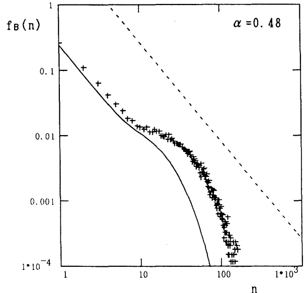
図7: バースト長分布 f_B(n) vs. n 。実線は理論式(20)、点線は f_B(n) \sim n^{-3/2} を表す。
