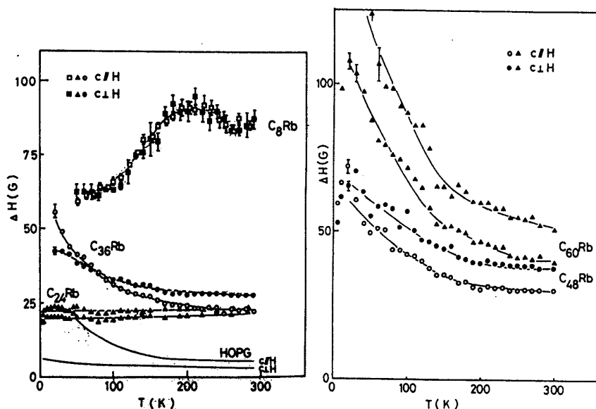
図3. 第1～第5ステージRb化合物の線幅の温度依存性
