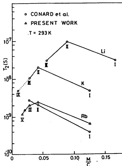
図2. アルカリ金属濃度とスピン緩和時間 ( \propto 1/\Delta H ) 添字はステージ
