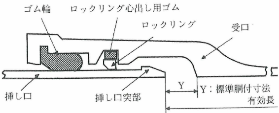
図3 離脱防止機能付きのダクトイル鋳鉄管
