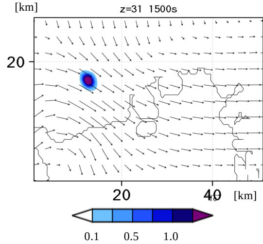
Fig. 12 実験5の水蒸気混合比を12%増した実験において発生した降水。ベクトルで水平風、陰影で雨水混合比 [\text{gkg}^{-1}] を示す。
