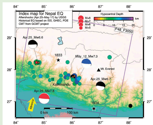
【図1】2015年ネパール地震とM5以上の余震の震央分布。深さに応じて色を変えて表示してある。★はM6以上の顕著な余震の震央。黒い★は、ネパールに被害をもたらした2つの地震の震央（位置は諸説ある）。発震機構解はMw6.6以上。紫色の四角は、「だいち2号」搭載合成開口レーダーの観測範囲を示す。黄色矢印は、インド・プレートのユーラシアプレートに対する運動方向を示す。緑色の■と、黒い▲は、それぞれカトマンズとエベレストを示す。
