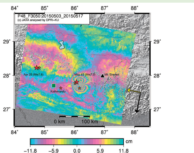
干渉画像。(左)2015年2月22日と地震後の5月3日の画像のペア、(右)5月3日と5月17日の画像の射出方向を示す。
