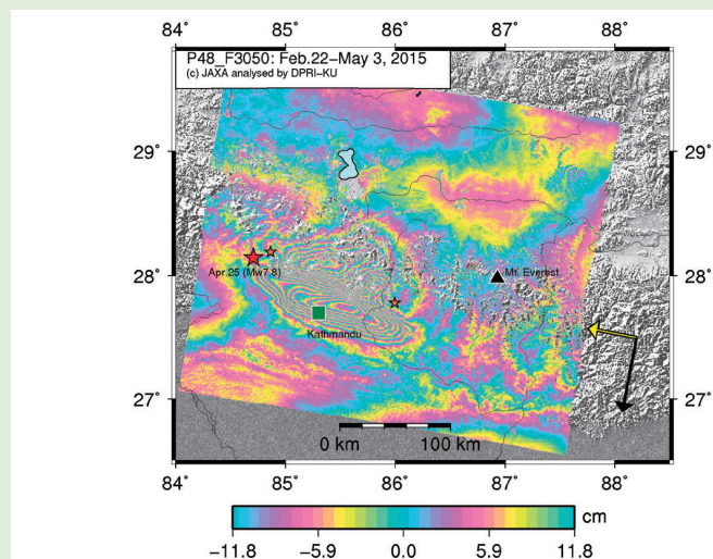
図2 「だいち2号」搭載合成開口レーダー画像のパス48フレーム3050のデータを用いて作成したのペア、から作成した干渉画像。図中 右下の黒と黄色の矢印は、それぞれ衛星の進行方向と電波
