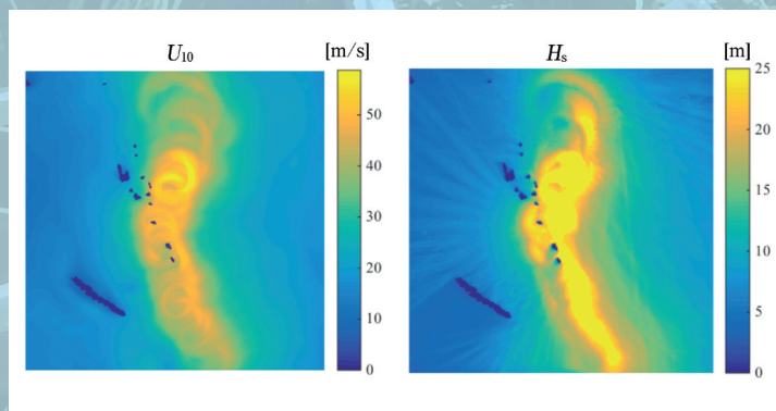
【図2】最大風速(左)と最大有義波高(右)
