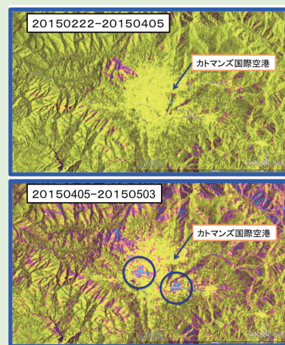
図3 「だいち2号」搭載合成開口レーダー画像を用いて作成したカトマンズ周辺のコヒーレンス画像。黄色→ピンク→青の順番で、コヒーレンスが低下する。(上)2015年2月22日と4月5日、の画像のペア、(下)4月5日と5月3日の画像のペアから作成したもの。カトマンズ市街では、地震前は全域でコヒーレンスが高い(黄色)。しかし、地震をはさむ期間のペアでは、大きくコヒーレンスが低下した地域があることがわかる。
