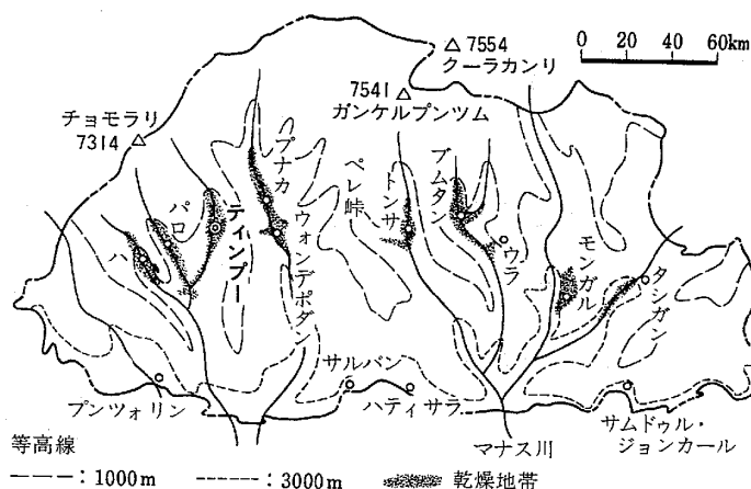
図4 山谷風による中央部乾燥地帯と標高出所 桑原（1978：120）
