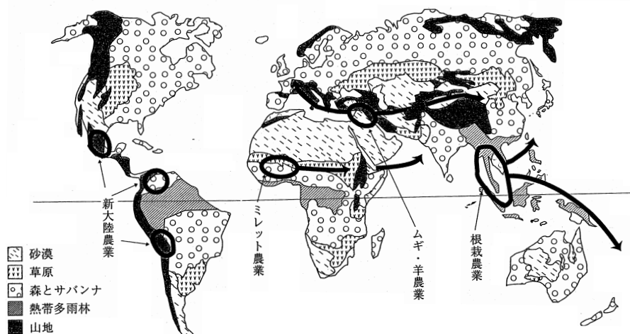
図2 世界の景観区と農業の4つの起源地 出所) 高谷 (2002: 14-15)
