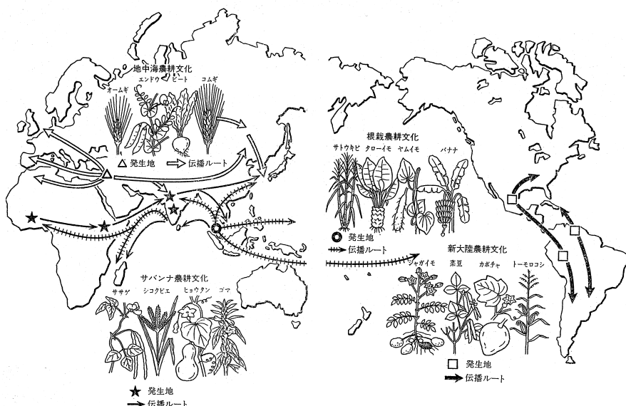
図1 4つの農耕文化基本複合 出所) 中尾 (1966 : vi-vii)
