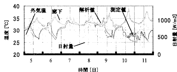
図 7 研究室・改修前の室温（日射透過率 0.8）
