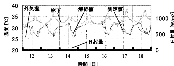
図 8 研究室・改修後の室温（日射透過率 0.4）
