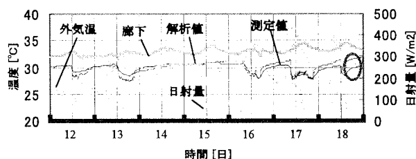
図 6 教員室・改修後の室温（日射透過率 0.4）
