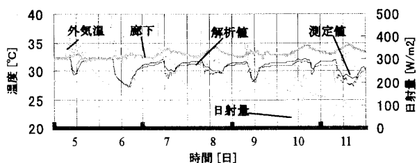
図 5 教員室・改修前の室温（日射透過率 0.8）
