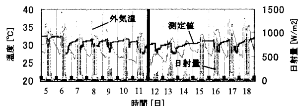
図2 教員室の室温実測値 (8月5日~8月18日)
