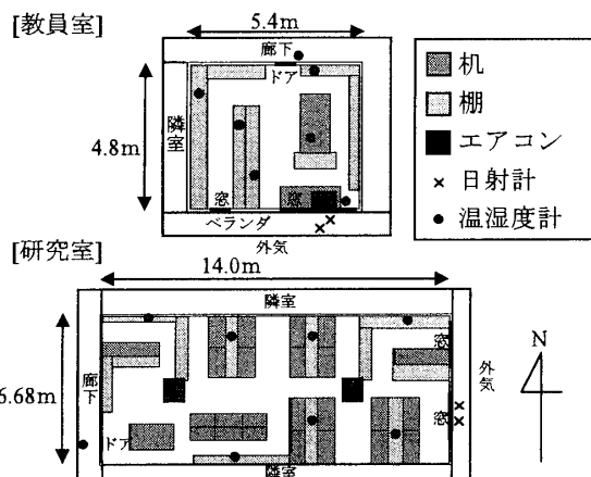
図1 教員室・研究室の平面図およびセンサー位置
