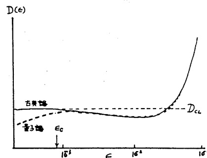
図-1 古典混合性の回復特性 ( \varepsilon : ほどほどに大)
