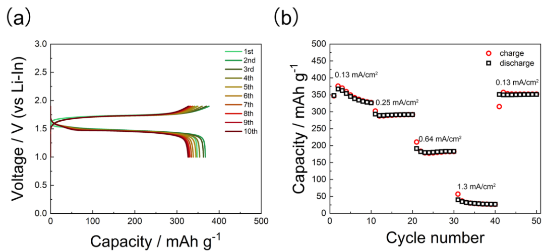
Figure 5.5. (a) Charge/discharge curves of \text{Li}_3\text{CuS}_2\text{-Li}_3\text{PS}_4 cathode, (b) cyclability of \text{Li}_3\text{CuS}_2\text{-Li}_3\text{PS}_4 .
