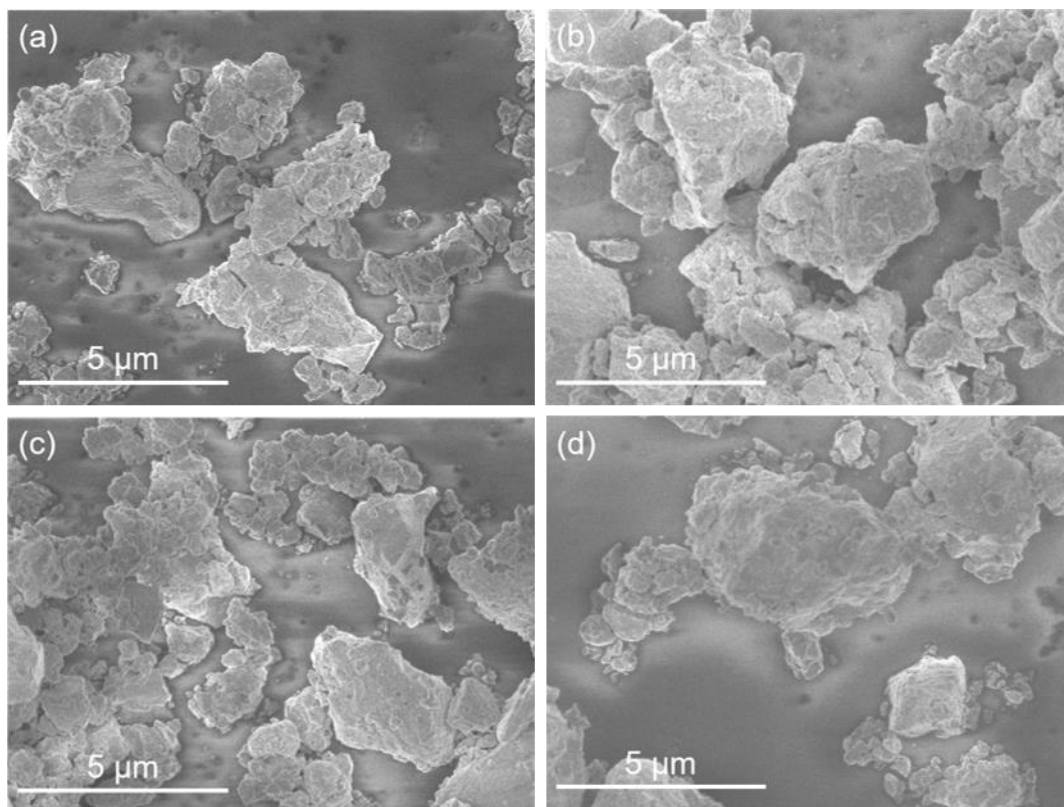
Figure 4.4. SEM images of (a) 100(0.75\text{Li}_2\text{S}-0.25\text{V}_2\text{S}_3) , (b) 95(0.75\text{Li}_2\text{S}-0.25\text{V}_2\text{S}_3)-5\text{LiI} , (c) 90(0.75\text{Li}_2\text{S}-0.25\text{V}_2\text{S}_3)-10\text{LiI} , and (d) 80(0.75\text{Li}_2\text{S}-0.25\text{V}_2\text{S}_3)-20\text{LiI} cathodes.
