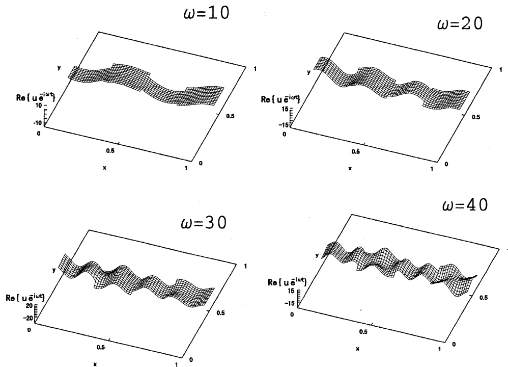
Figure 2: 異なる波数 \omega についての数値計算結果
