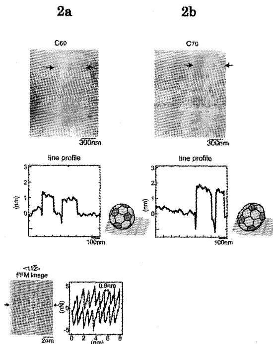
図 2 グラファイトの上の C 60 膜と C 70 膜 AFM 像 (凹凸像)。図の中間に、矢印で示されたところのラインプロファイルが与えられている。C 60 膜の厚さは約 1nm である。下図の C 60 単層膜の高分解摩擦力像は約 0.9nm の周期を与えており、これは C 60 単層膜の \langle 11\bar{2} \rangle 方位に沿ってジグザグ運動していることを示している。C 70 膜の高さは 2nm で 2 層膜であることを示す。
