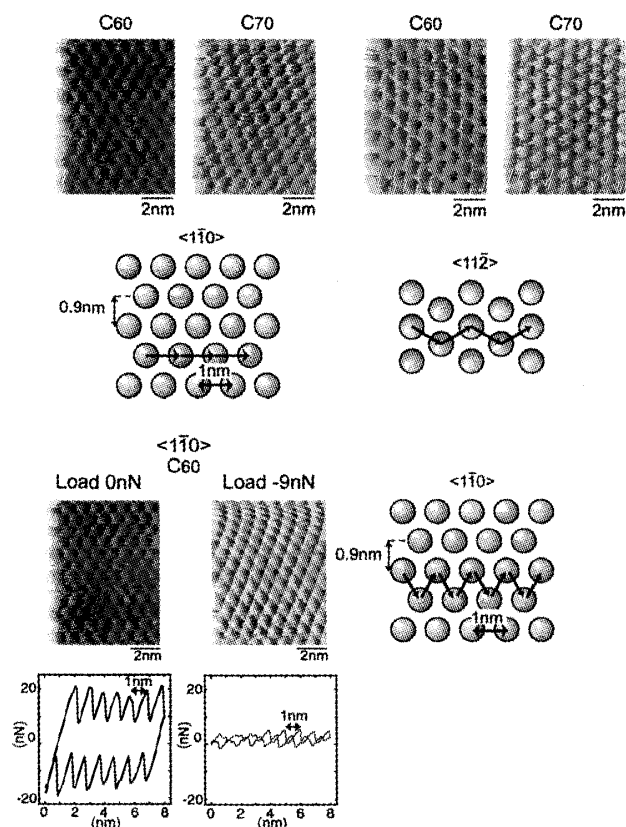
図4 C_{60} 膜と C_{70} 膜の(111)面からの高分解摩擦力像。
