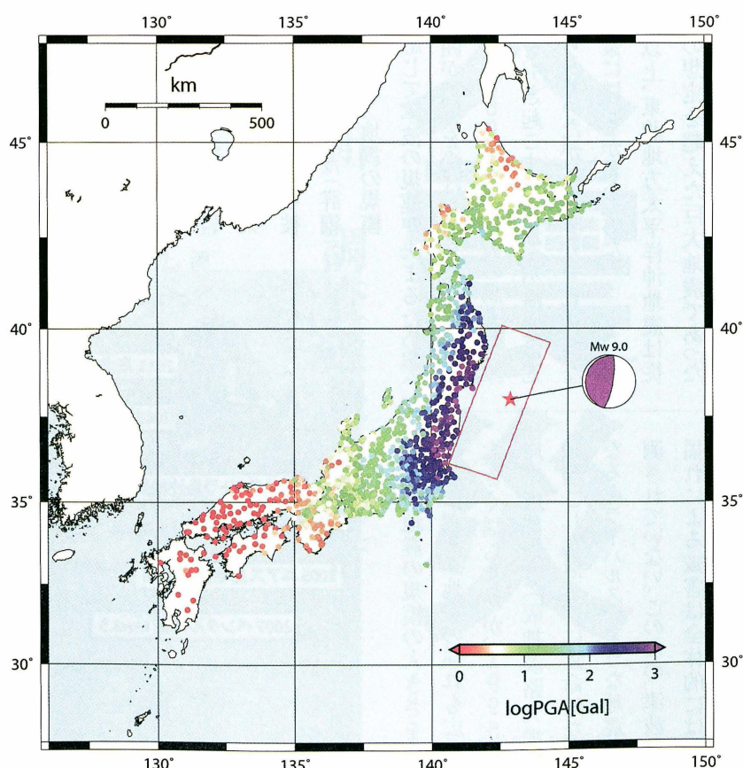
図2 最大加速度の分布と震源断層のおおよその位置、震源メカニズム
