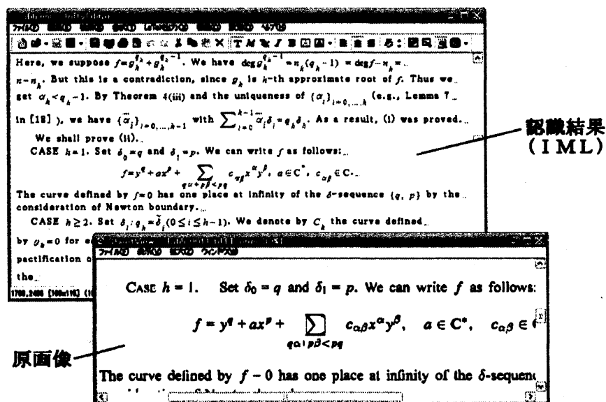
図 4: 認識結果の InfyEditor での確認・編集
