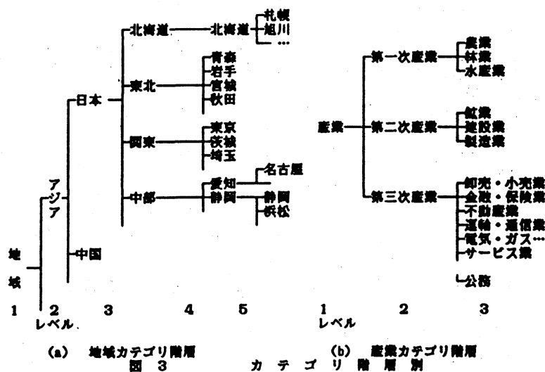
図2 生成規則例
