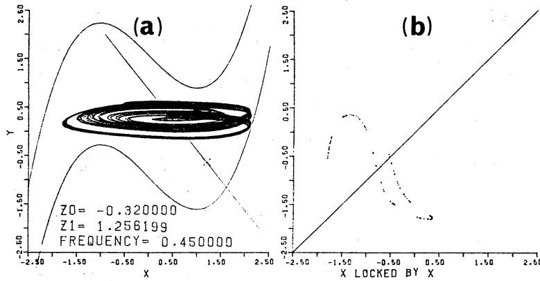
図7 chaotic解 (a): x は平面上の軌道, (b): x の極小値に関するロレンツ・プロット中
