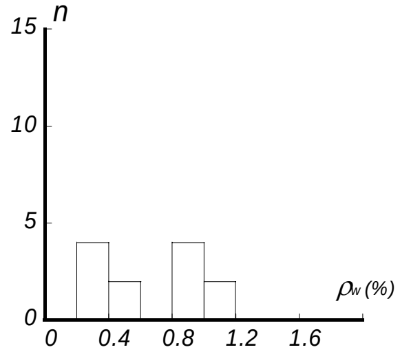
(d) Shear reinforcement ratio
