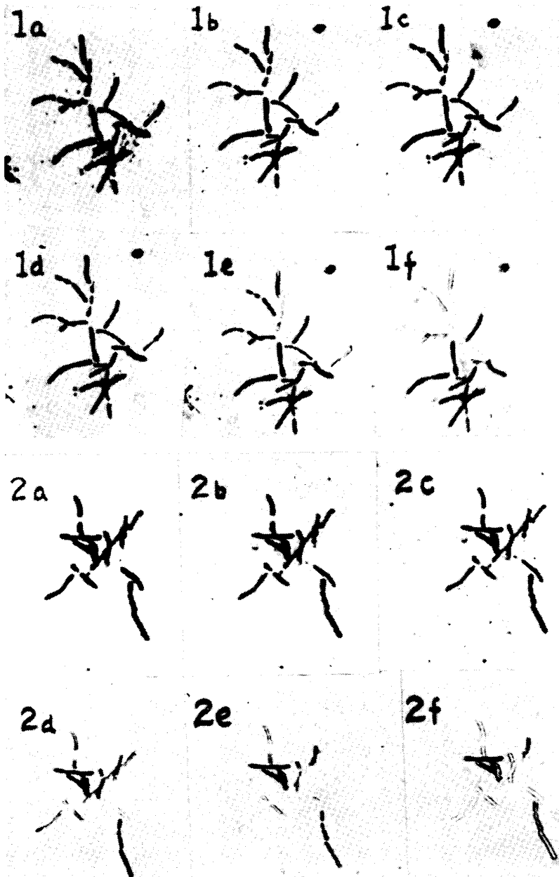
Fig. 1. 2. 石炭酸フクシン加温染色後 70%アルコール (a), 0.3% (b), 1% (c), 3% (d), 10% (e), 30% (f) HCl アルコールで脱色した鳥型結核菌の microcolony.
