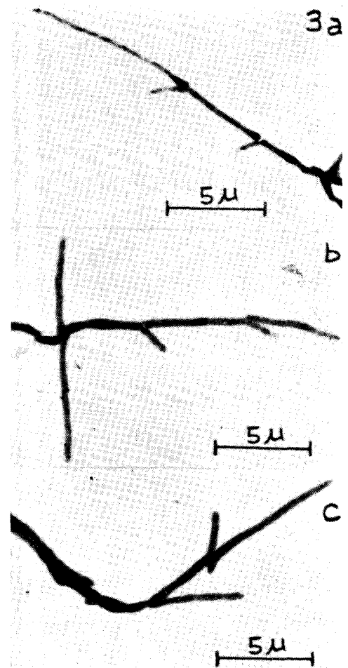
Fig. 3. a, b, c. 培養5日のスメグマ菌の電顕写真。樹枝状発育を示す。
