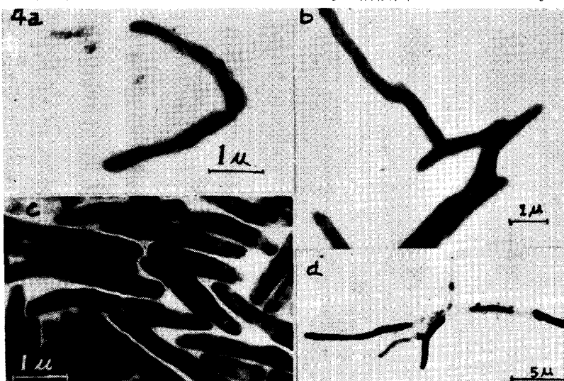
Fig. 1. 2. 石炭酸フクシン加温染色後 70%アルコール (a), 0.3% (b), 1% (c), 3% (d), 10% (e), 30% (f) HCl アルコールで脱色した鳥型結核菌の microcolony.
