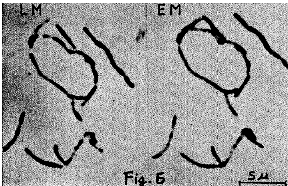
Fig. 6. 鳥型結核菌の陳旧培養のmicrocolonyの染色像並びに電顕像 LM. Ziehl-Neelsen 染色光学顕微鏡写真 EM. 同電顕写真
