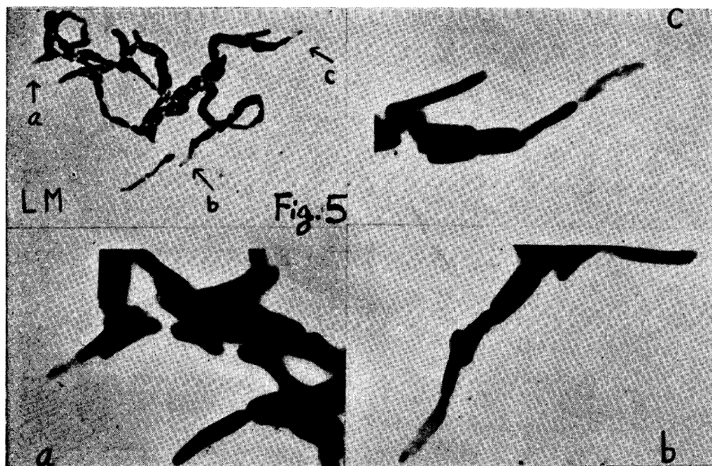
Fig. 5. 鳥型結核菌の初期培養のmicrocolonyの染色像並びに電顕像 LM. Ziehl-Neelsen 染色光学顕微鏡写真 a. b. c. 同電顕写真
