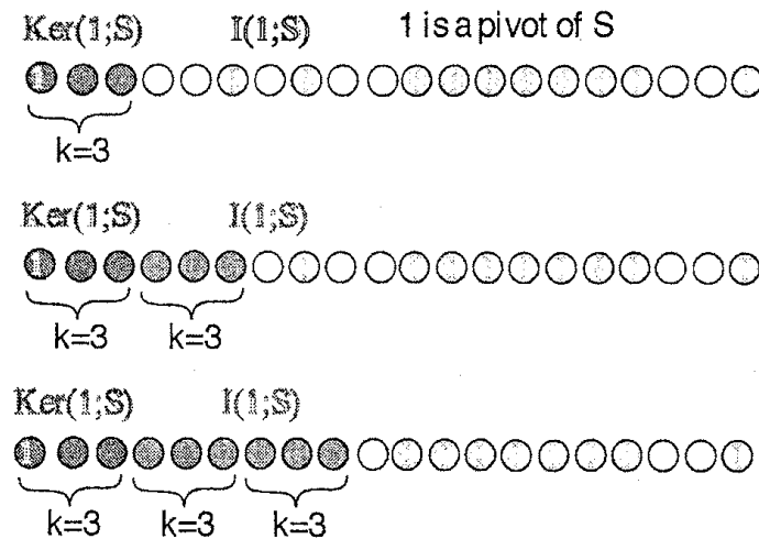
FIGURE 13. I(1; S) の再生
