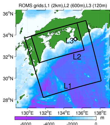
図-5 ROMSによる3段ネスト領域と水深分布（カラー）。黒枠は外側から、ROMS-L1（水平解像度 2 km）、L2（同 600 m：瀬戸内海全域モデル）、L3 領域（同 120 m：田辺湾モデル）の境界を示している。
