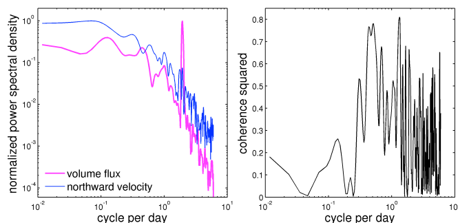
図-7 (左) 湾口通過体積フラックス（マゼンタ）と田辺湾沖合における北向き表層流速（青）の無次元パワースペクトル，（右）両者のコヒーレンス。
