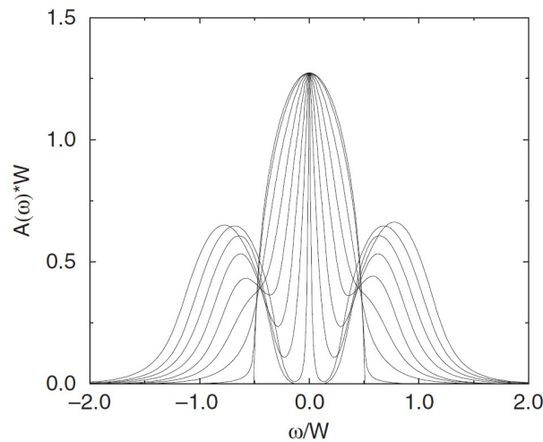
図 12: 動的平均場理論によるハバード模型の一粒励起スペクトル (ハーフフィリング)。状態密度はバンド幅 W の半円形。不純物ソルバーは NRG 法。 U の値は U/W = 0 から 1.6 まで 0.2 刻みである。文献 [27] より。
