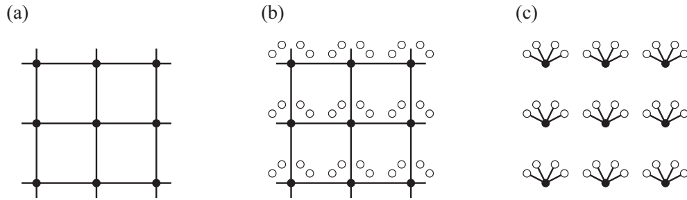
図 19: 自己エネルギー汎関数理論の概念図。(a) 元の格子模型。黒丸は相関のある格子点。(b) 元の格子模型と等価な模型。白丸は相互作用の無い格子点 (bath)。(c) 参照系。文献 [53] より。
