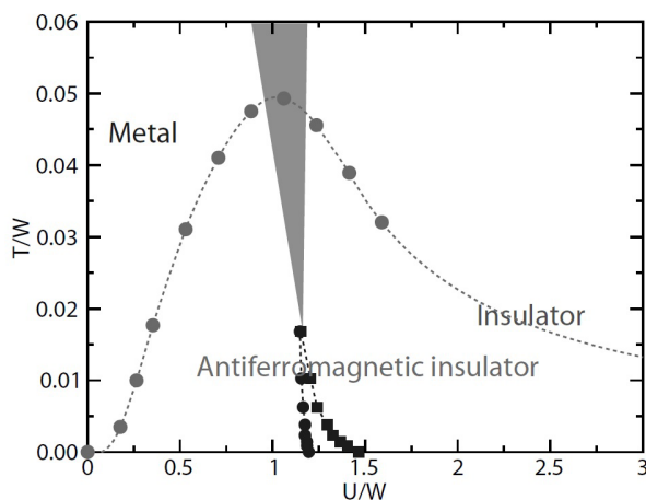
図 13: 動的平均場理論によるハバード模型の反強磁性相図（ハーフフィリング）。低温の四角は反強磁性を無視した計算で得られたモット転移（1 次転移）で、影の部分は金属と絶縁体のクロスオーバー領域を表す。立方格子上的最近接ホッピングを考慮した模型でバンド幅 W = 12t で規格化している。不純物ソルバーは NRG 法。文献 [28] より。
