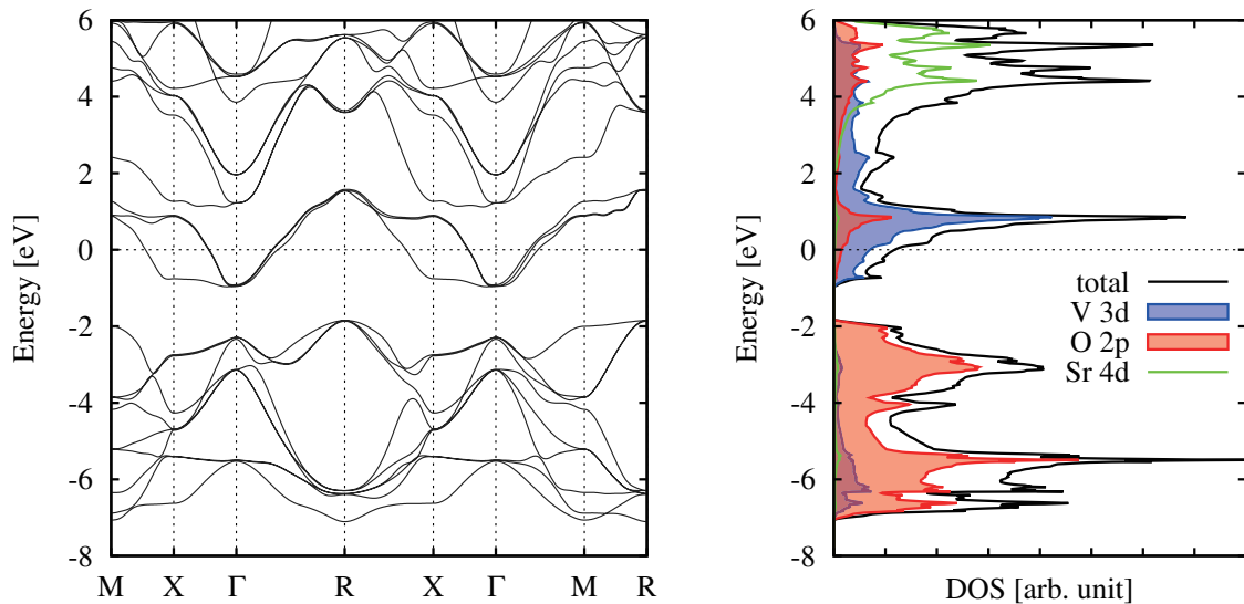
図 3: ペロブスカイト構造を持つ化合物 \text{SrVO}_3 のエネルギーバンド分散 (左) と状態密度 (右)。LDA による計算。フェルミ準位 E_F = 0 付近の 3 つのバンドは V の 3d\text{-}t_{2g} 軌道、フェルミ準位以下の 9 つのバンドは O の 2p 軌道である。
