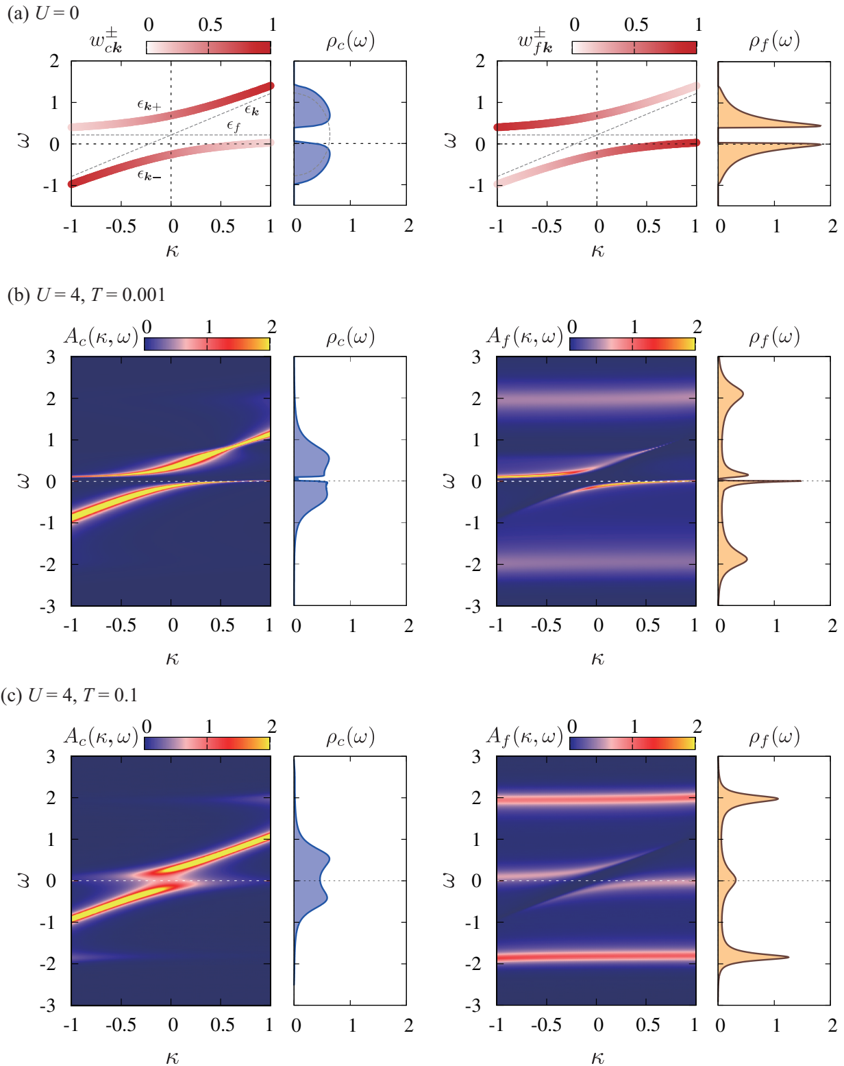
図 14: (a) U=0 の周期アンダーソン模型のエネルギー分散を「波数」 \kappa \equiv \epsilon_{\mathbf{k}} の関数として表した図。左が伝導電子 c、右が f 電子。色の濃さは重み w_\alpha^\pm を表す。点線は混成がない場合のエネルギー分散。ベーテ格子上の強束縛バンド（状態密度はバンド幅 2D の半円形）を考えている。パラメータは D=1 として、 V^2=0.22 , n=1.9 である。(b),(c) は U=4 の場合の動的平均場理論による一粒子励起スペクトル A_\alpha(\kappa, \omega) と状態密度 \rho_\alpha(\omega) 。ソルバーは CTQMC 法。(b) T=0.001 , (c) T=0.1 。
