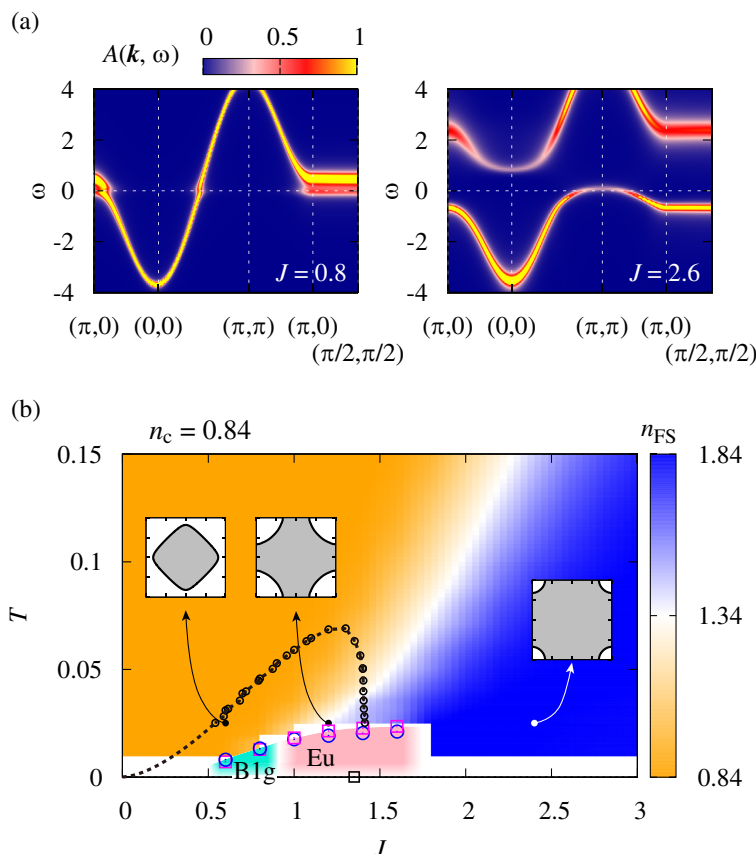
図 21: デュアルフェルミオン法による 2 次元正方格子上の近藤格子模型における (a) 一粒子励起スペクトルと (b) 超伝導相図 [59]。伝導電子数 n_c = 0.84 のハーフフィリング近傍。 B_{1g} と E_u はそれぞれスピナー重項の d_{x^2-y^2} 波と p 波の対称性を持つ超伝導。強度プロットはフェルミ面の囲む体積によって定義される電子数 n_{FS} を表す。丸と点線は反強磁性相の目安を表す (ハーフフィリングの場合)。図は文献 [7] より。
