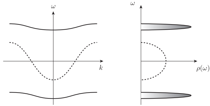
図 8: ハバード I 近似によるエネルギーバンド（左）と励起スペクトル（右）。点線は相互作用がない場合（ \Sigma = 0 ）に対応。実線は重み 1/2、点線は重み 1 である。
