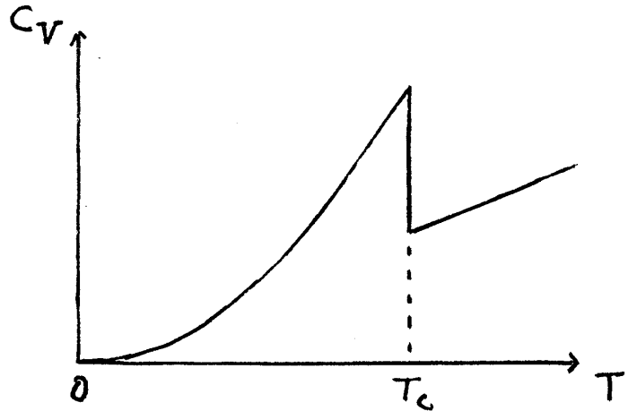
第 4-2 図 定積比熱 C_V の温度依存性
