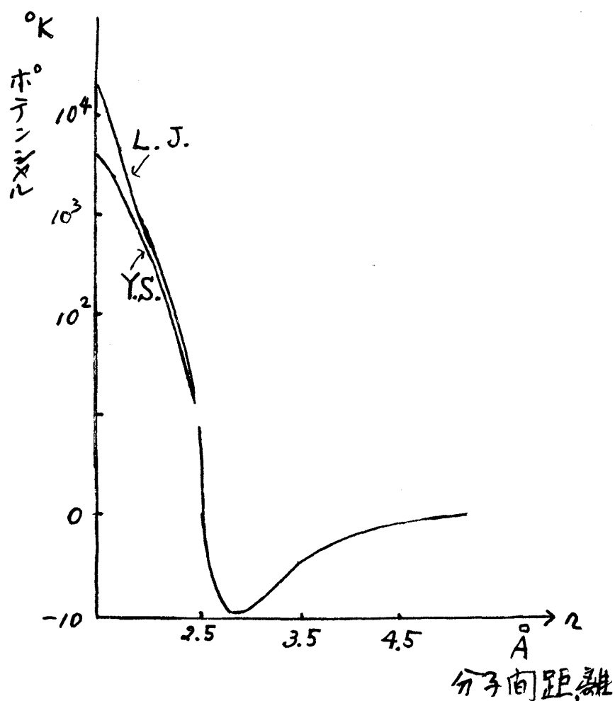
第 2-1 図 ^3\text{He} 粒子間に働く裸のポテンシャル
