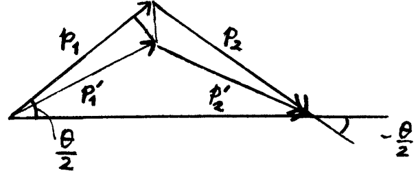
第 9-1 図 散乱粒子の運動量関係図
