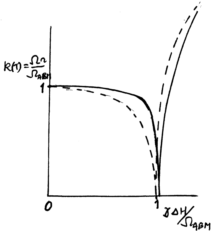
第 12-1 図 A 相での共鳴振動数 \Omega_r と input \gamma\Delta H との関係。実線は緩和効果のある場合、点線は無い場合。
