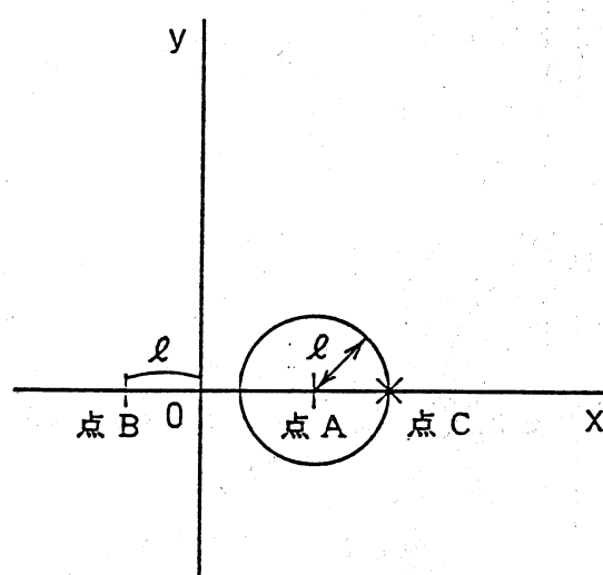
(b) B < 0 の場合
