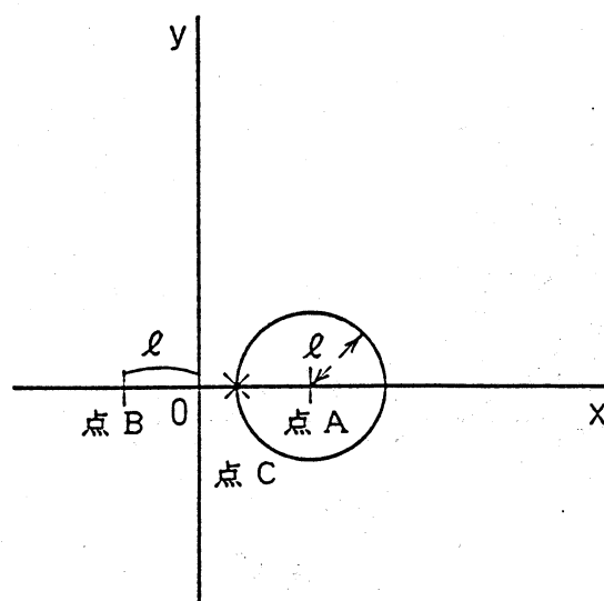
(b) B < 0 の場合
