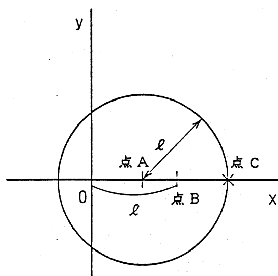
(a) B > 0 の場合
