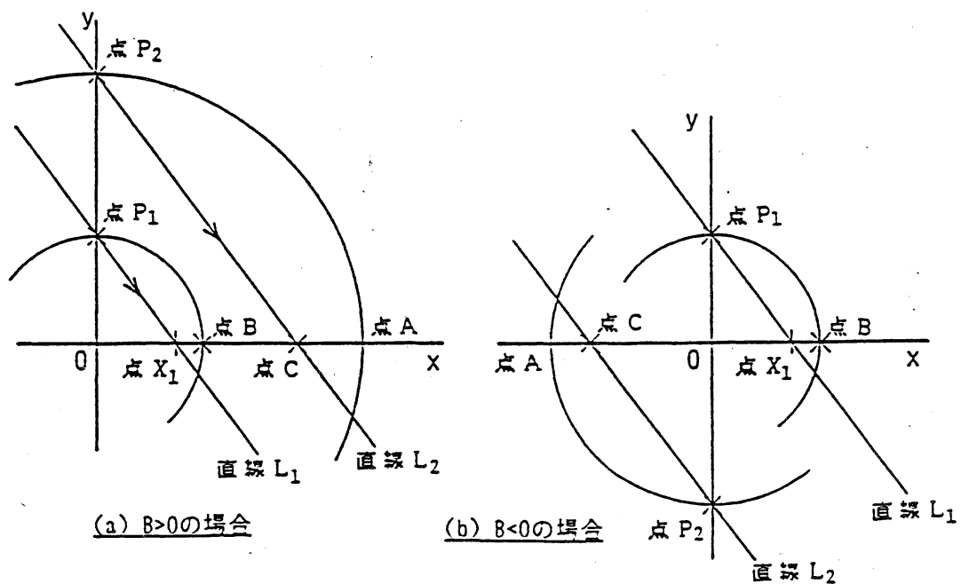
図1.4 C = A / B の作図
