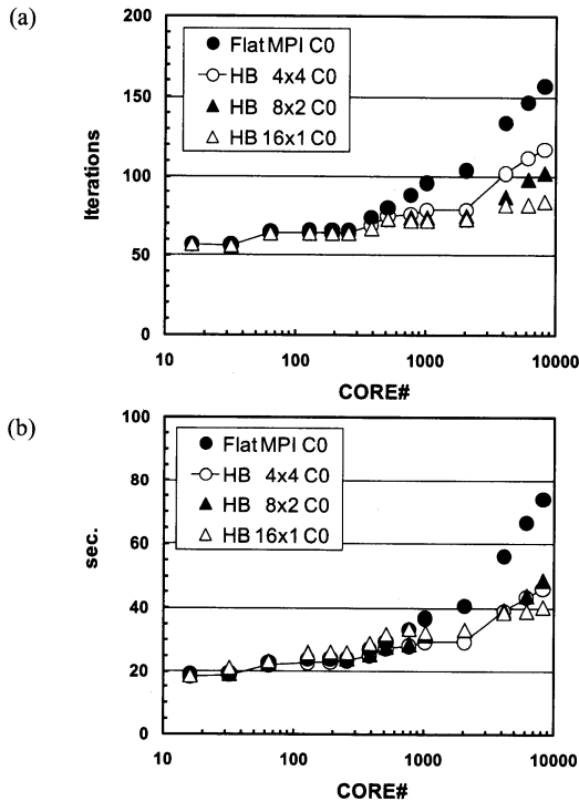
図 14 MGCG 法の計算性能 (C0) ((a) 反復回数, (b) MGCG ソルバー計算時間) (最適化されたソルバーを適用, CM-RCM(2), 16~8,192 コア, T2K (東大)) (Weak Scaling, 262,144 セル/コア, 最大問題規模: 2,147,483,648 セル) (不均質多孔質媒体中の三次元地下水流れ)
