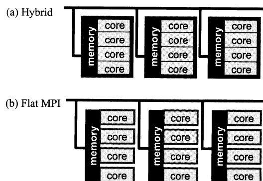
図1 並列プログラミングモデルの例
