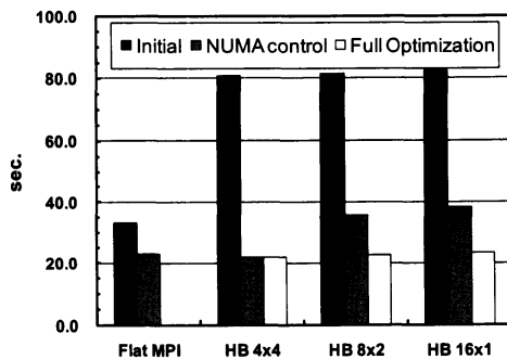
図 12 MGCG 法の計算性能と最適化の効果 (MGCG ソルバー計算時間) (CM-RCM(2), 16,777,216 セル, T2K (東大), 64 コア) (不均質多孔質媒体中の三次元地下水流れ) (■Initial: 初期状態, ■NUMA control: 実行時の最適な NUMA control の適用, □Full Optimization: NUMA Control, First Touch Data Placement, 連続データアクセスのための再データ配置を全て適用した場合)
