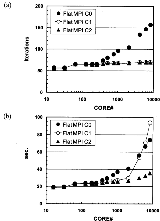
図 15 MGCG 法の計算性能 (Coarse Grid Solver の効果: C0, C1, C2) ((a) 反復回数, (b) MGCG ソルバー計算時間) (最適化されたソルバーを適用, CM-RCM(2), 16~8,192 コア, T2K (東大), Flat MPI) (Weak Scaling, 262,144 セル/コア, 最大問題規模: 2,147,483,648 セル) (不均質多孔質媒体中の三次元地下水流れ)
