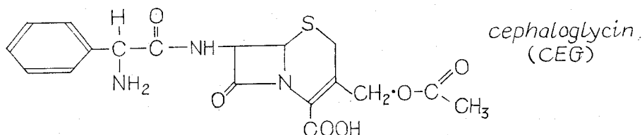
Fig. 1 構 造 式
