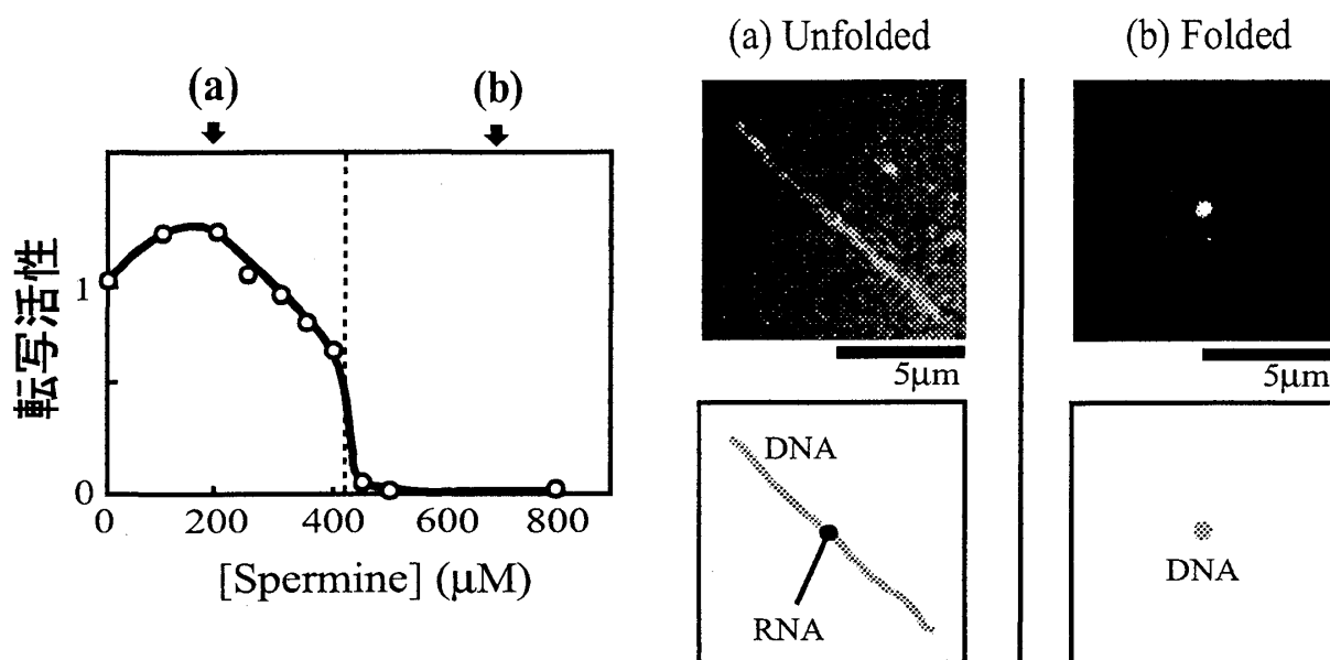
図 1: (左)DNA アンサンブルにおける凝縮剤濃度変化と転写活性の相関 [1]。(右) 転写反応後、ガラス基板上に引き伸ばされたコイル状態 (a) とグロビュール状態 (b) の DNA。コイル状態の DNA 分子上にのみ、合成された mRNA が観察された。
