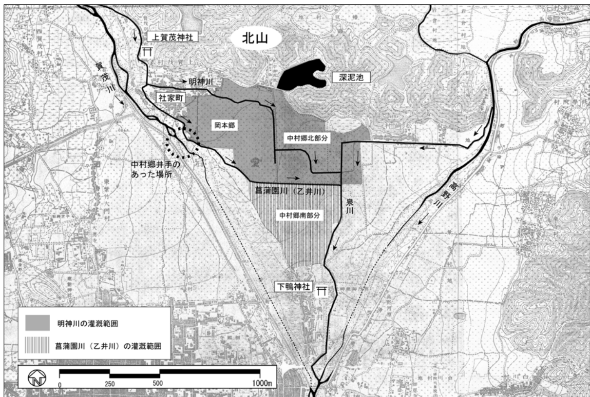
図-1 中世の上賀茂神社領岡本郷と中村郷への灌漑水路 (須磨千穎『賀茂六郷境内諸郷の復元的研究』内「[1]宝徳三年岡本郷地からみ帳記載田地復元図」 「[4]宝徳三年中村郷地からみ帳記載田地復元図」を参照し『明治22年仮製2万分の1地形図』上に筆者作成)
