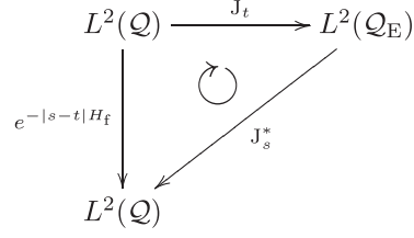
Figure 3. e^{-|s-t|H_f} の分解
