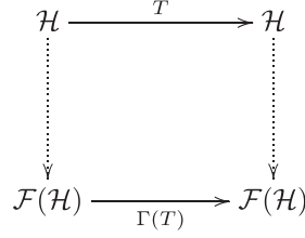
Figure 1. ファンクター \Gamma
