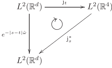
Figure 2. e^{-|s-t|\hat{\omega}} の分解
