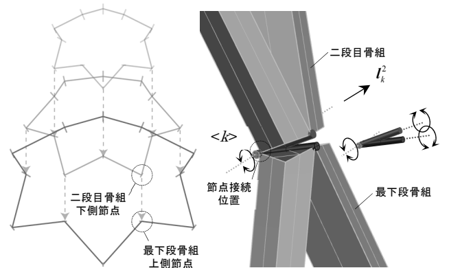
図 14 ドーム型骨組の構成方法
