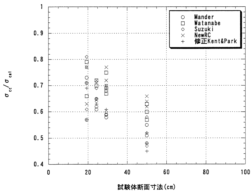
図 5-2 横拘束タイプの最大耐力の算定結果と試験体寸法の関係
