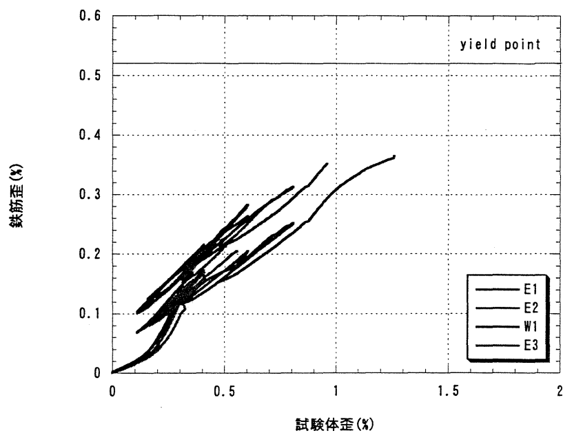
図 4-11 1.5%タイプの試験体歪-鉄筋歪関係
