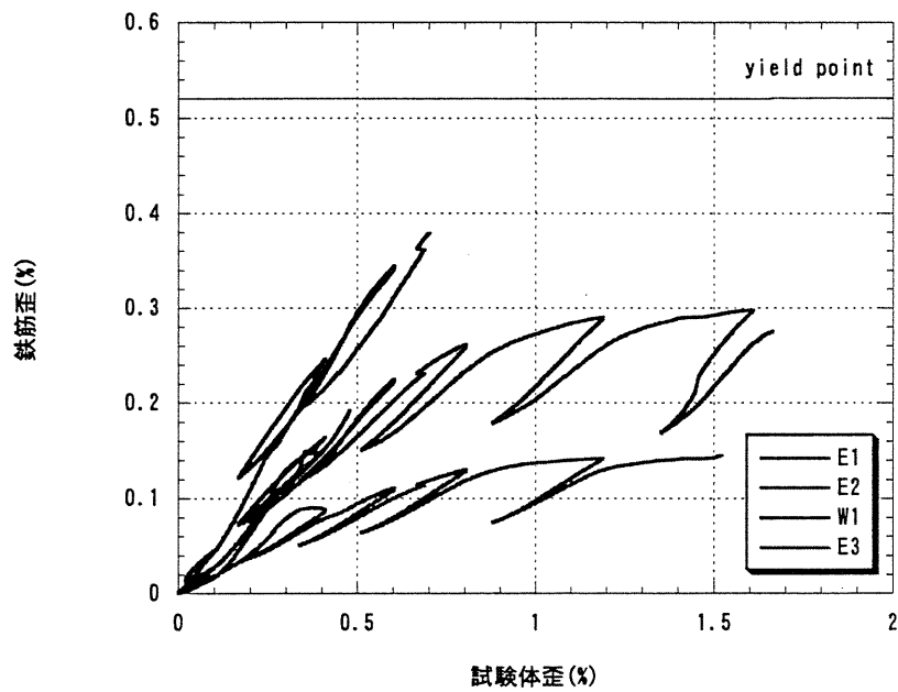
図 4-12 2.0%タイプの試験体歪－鉄筋歪関係
