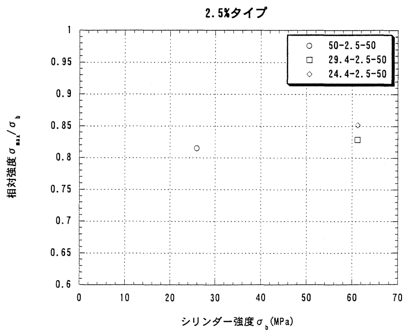
図 4-1 コンクリート強度の影響
