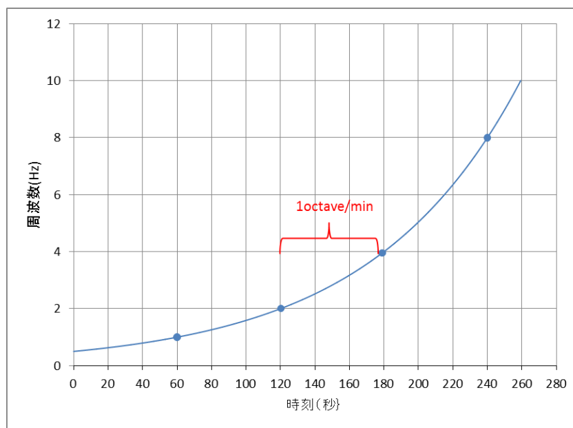
図 3 周波数遷移
