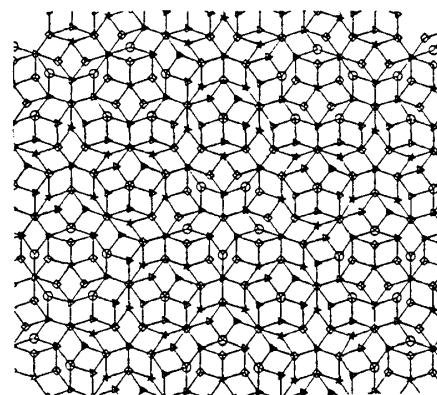
図4. Penrose図形のvertexの分類.
