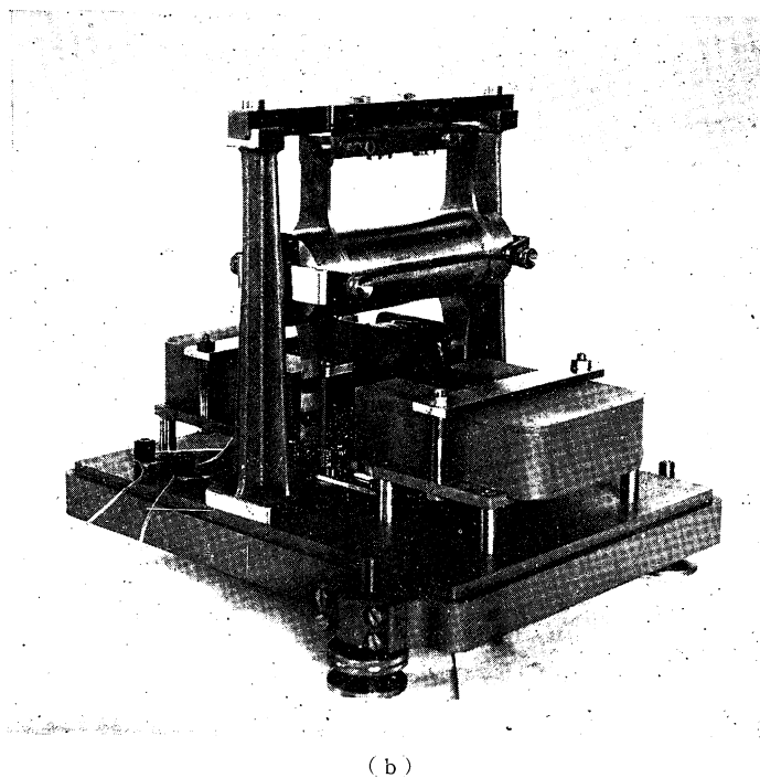
Fig. 3. (a), (b) Horizontal seismometer of A-2 ( R_2 )-type.
