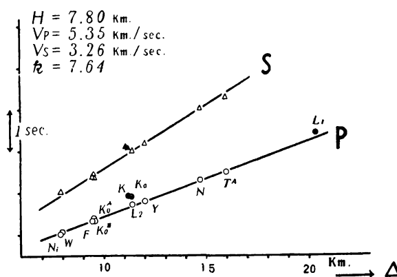
Fig. 7. Time-distance cuaves. (No. 217)
