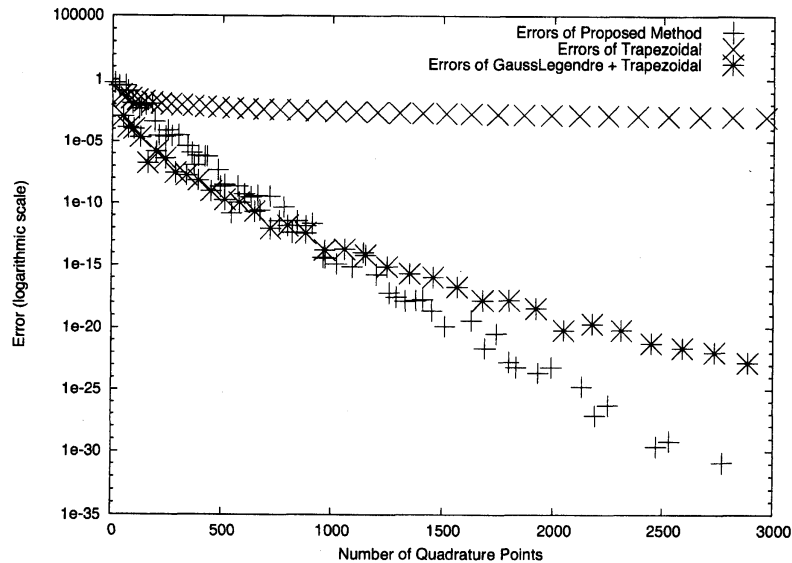
図 4: 球面上の積分則の節点数と誤差
