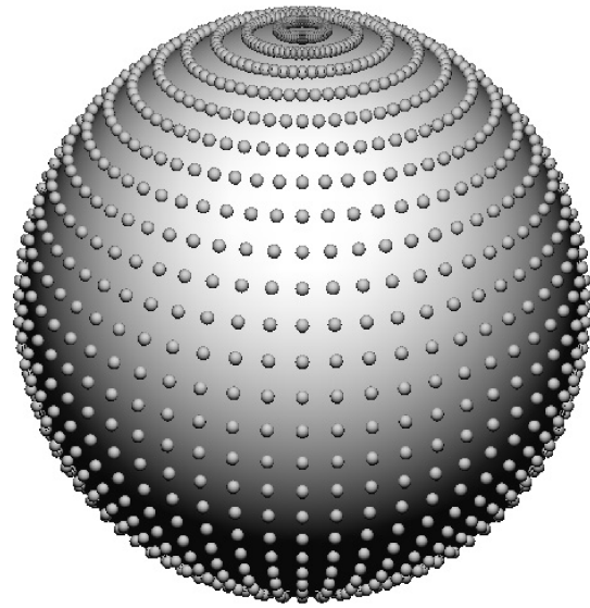
図 6: 緯度方向に 30 点の Gauss-Legendre 則, 経度方向に台形則の場合の標本点, 点数は 1800
