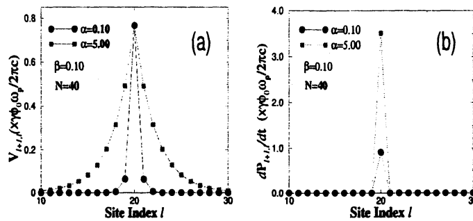
図 6: (a) \alpha = 0.10 及び \alpha = 5.00 での一つの回転局在モードにおける電圧分布。接合（振り子）数は N = 40 であり、周期境界条件が採用されている。(b) 一つの回転局在モードにおける \frac{dP_{i,i+1}}{dt} の分布。
