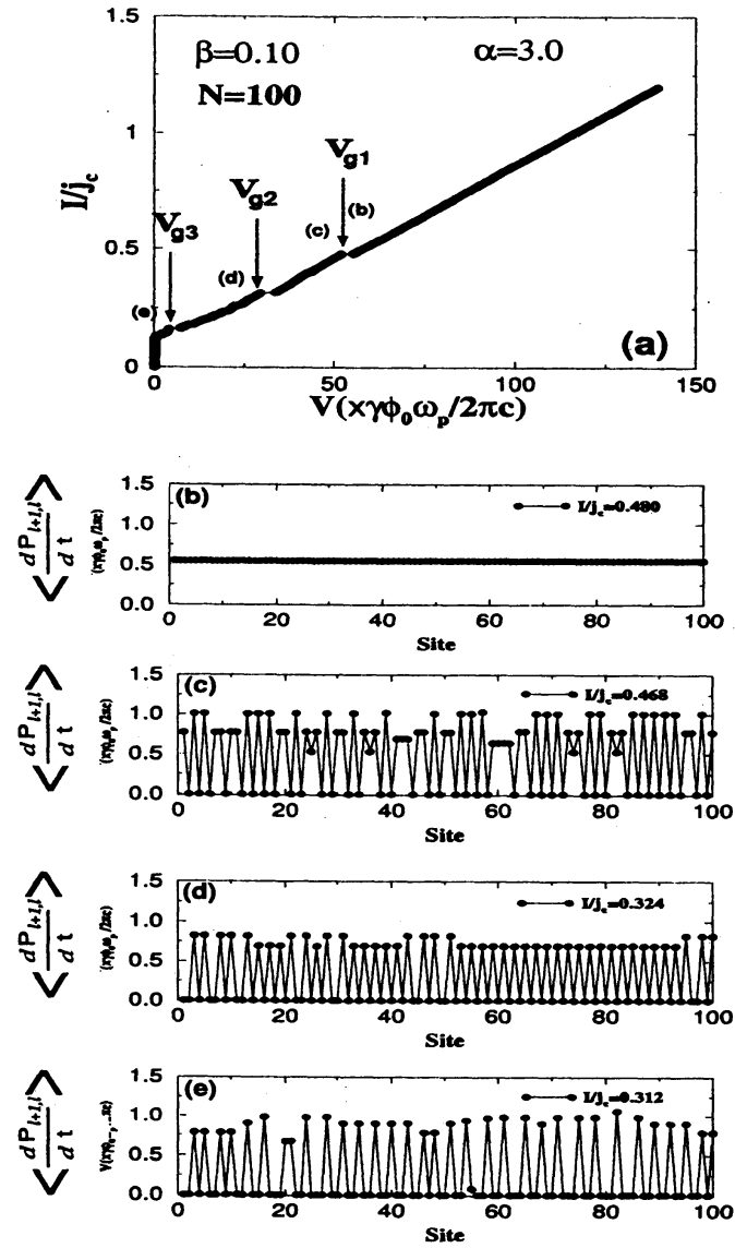
図 8: \alpha = 3.0 の電流電圧特性。以下、平均回転速度 \langle \frac{dP_{\ell+1,\ell}}{dt} \rangle の空間分布が示されている。各々 (b) V_{g1} 以上, (c) V_{g1} 以下 (d) V_{g2} 以下 (e) V_{g3} 以下で測定された空間分布である。
