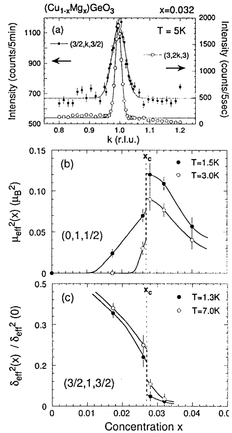
図 10: (a) x = 0.032 の試料における (3/2, k, 3/2) の超格子ピーク。白丸は測定分解能を示すために載せた (3, 2k, 3) のブラッグピーク。超格子ピークの線幅は明らかに分解能より広がっている。(b) \text{Cu}_{1-x}\text{Mg}_x\text{GeO}_3 の有効磁気モーメントの自乗。(c) \text{Cu}_{1-x}\text{Mg}_x\text{GeO}_3 の格子ひずみの自乗。文献 [34] より。
