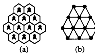
図 2: 無線通信局の配置 (a) と対応するグラフ (b)
