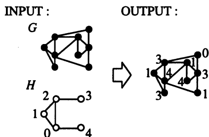
図 1: COLRAC の問題例
