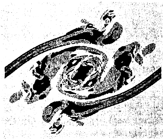
図 6 混合層の局所トポロジー分布 黒い部分；不安定焦点・渦収縮、 灰色部分（背景を除く）；安定焦点・渦伸張。 原図はカラーであり赤と緑の部分があるがごく少ない空間を占めている。
