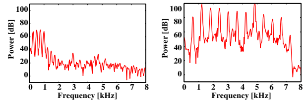
(a) 平静音声 (b) 叫び声 図1 平静音声と叫び声の対数パワースペクトル
