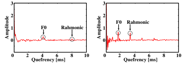
(a) 平静音声 (b) 叫び声 図2 平静音声と叫び声のケプストラム
