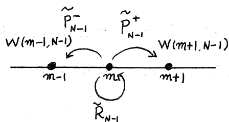
図2. W(m \pm 1, N-1) で制御されたジャンプ。
