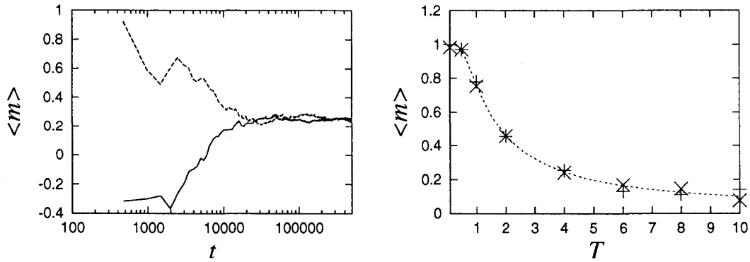
図 3: 同じ温度の磁場中 1/2-スピン 2 個の系。(左) 2 つのスピンの期待値の時間依存性 ( T = 4 の場合)。スピンの期待値が収束するのが見える。(右) 2 個のスピンの期待値 (+, ×) とその温度依存性。理論的期待値 \tanh(1/T) (点線) との一致が良いことがわかる。
