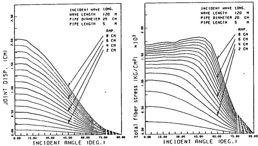
(1) longitudinal wave
