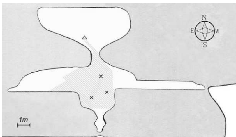
図 2 白浜町鴨居海岸のタイドプールに 2007 年に出現した 3 個体のオニヒトデの半月間の移動範囲 (斜線部)。× : 3 個体の初出現場所 (5 月 16 日)。△ : 1 個体が初めて移動した場所 (5 月 18 日)。図の白抜き部は外海を、黒い部分は岩礁を示す。
