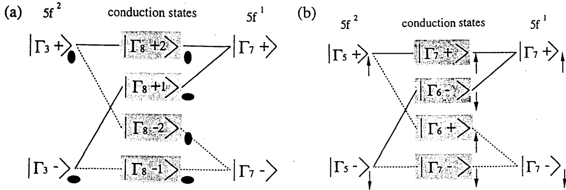
図 3: 立方対称 (a) および正方対称 (b) の f^2 配位における TCKE 機構の概念図。 f^2 安定配位の非クラマース二重項 (立方対称では \Gamma_3 , 正方対称では \Gamma_5 ) と中間励起 f^1 配位のクラマース二重項 \Gamma_7 間の遷移は、陰影部に示した伝導部分波状態との混成を通じてのみ起こる。実線と破線で示した各チャンネルの摂動から得られる有効結合定数は等しい値となる。矢印と楕円はそれぞれスピンと四重極を模式的に表している。
