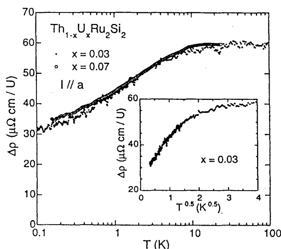
図 9: \text{Th}_{1-x}\text{U}_x\text{Ru}_2\text{Si}_2 ( x \leq 0.07 ) a 軸電気抵抗における混入 U の寄与.
