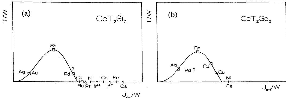
図 2: CeT 2 X 2 ( T : 遷移金属元素; (a) X = \text{Si} , (b) X = \text{Ge} ) 系における磁気転移温度の混成強度計算値に対するプロット [26]. 記号 +, □, △ はそれぞれ T = 3d, 4d, 5d 遷移金属元素に対応する。磁気転移を示さない物質は横軸上に記してある。
