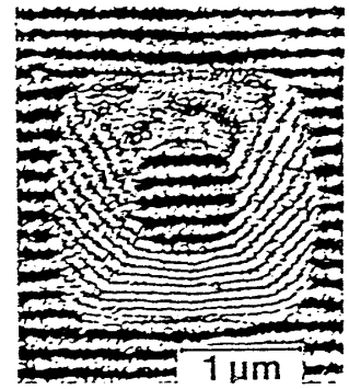
(b) 電子線の干渉写真
