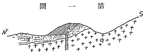
鍋山火山相像斷面圖
